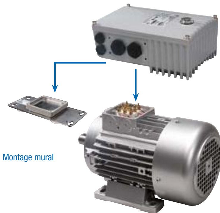
Montage moteur
