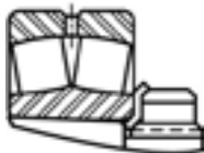
Figure 11. Montage sur arbre conique
