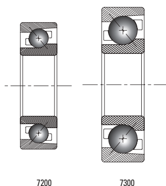
Figure 17. Séries de roulements à billes à contact oblique à une rangée.
