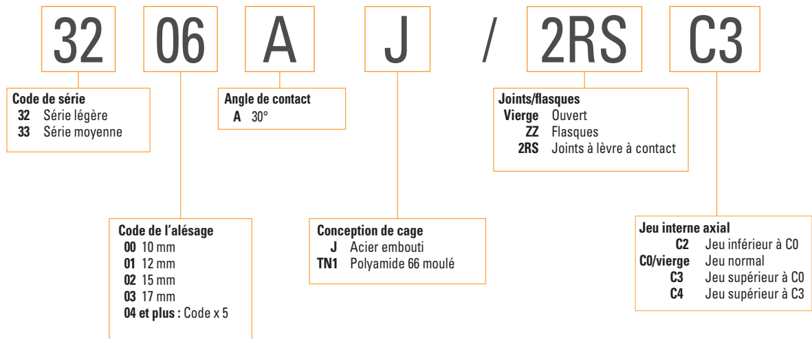
Figure 18. Nomenclatures des roulements à billes à contact oblique à deux rangées.
