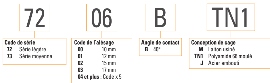
Figure 15. Nomenclature des roulements à billes à contact oblique à une rangée de conception standard.
