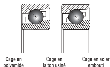
Figure 1. Variantes de cage : une rangée
