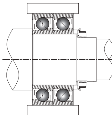
Figure 8. Montage en tandem (DT).
