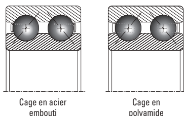
Figure 2. Variantes de cage : deux rangées
