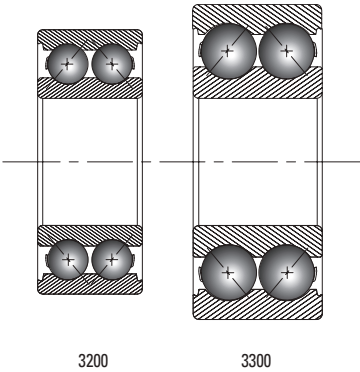
Figure 19. Séries de roulement à billes à contact oblique à deux rangées.
