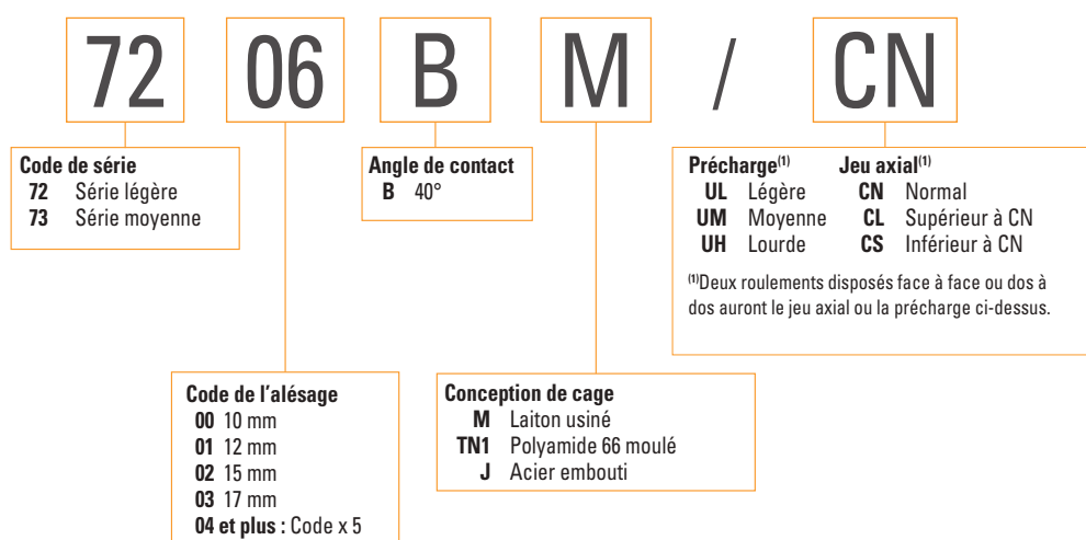
Figure 16. Nomenclature des roulements à billes à contact oblique à une rangée et pour appairage universel
