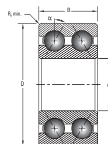
Figure 9. Conception de roulement à deux rangées.
