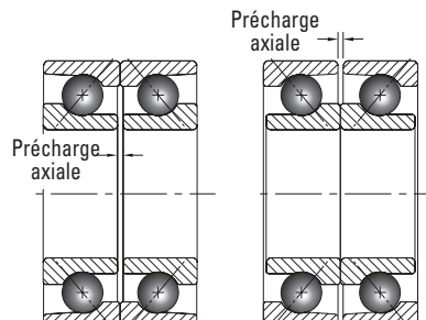
Figure 12. Précharge axiale pour les roulements à appairage universel
