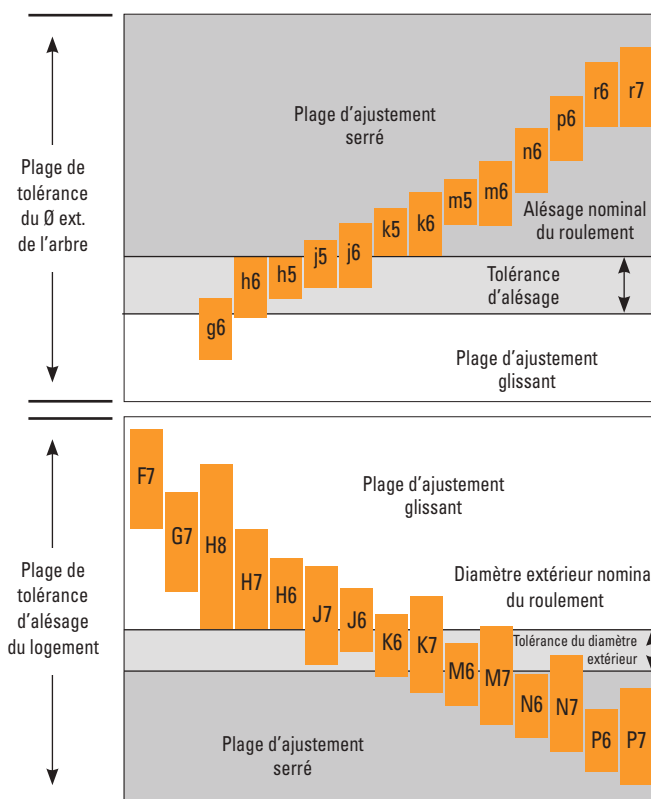
Figure 14. Sélections d'ajustement pour l'arbre et le logement du roulement.
