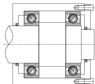
Figure 5. Deux roulements à billes à contact oblique à une rangée en montage DF standard.
