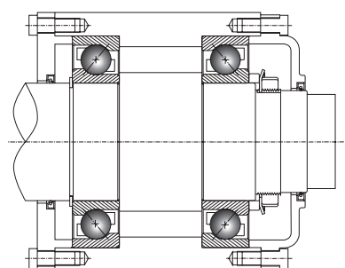
Figure 4. Deux roulements à billes à contact oblique à une rangée en montage DB standard.
