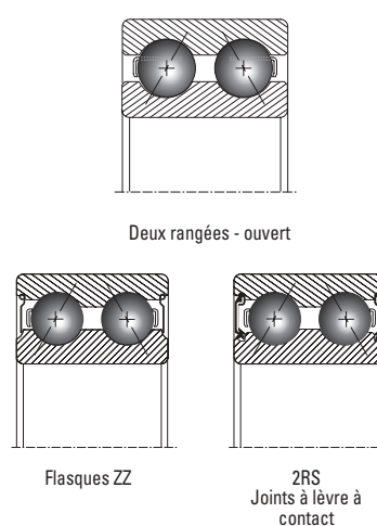
Figure 10. Configurations de roulements à deux rangées
