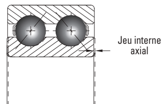
Figure 13. Jeu axial des roulements à deux rangées.
