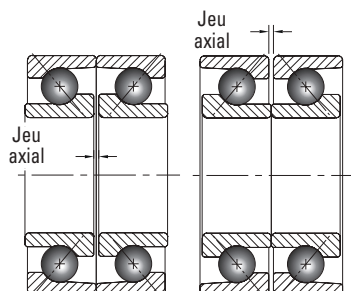
Figure 11. Jeu axial pour les roulements à appairage universel
