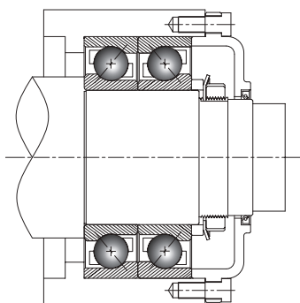
Figure 6. Montage dos à dos DB.
