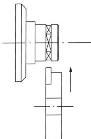
Fraisage en plongée
