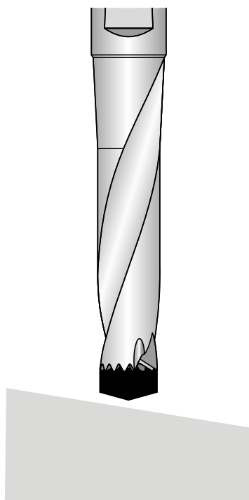
Entrée ou sortie sur surface inclinée
