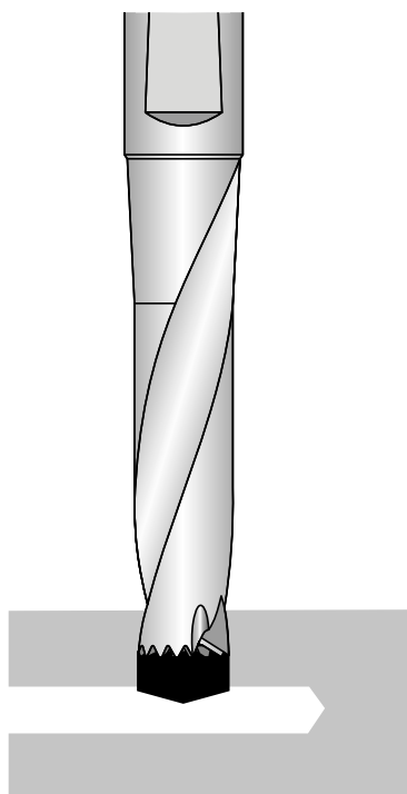
Perçage d'un trou sécant existant
